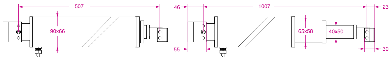
lunghezza attuatore chiuso / length of the closed strut
