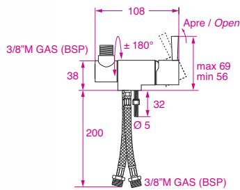
Maniglia / Handle SPM11LEVA MIN.
