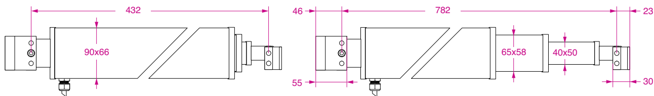
lunghezza attuatore esteso / length of the extended strut
