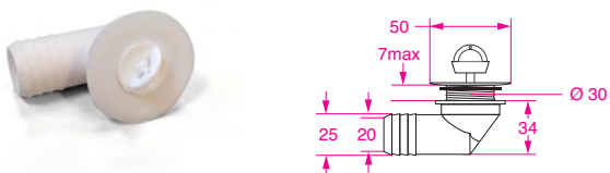
PIEL25F Peso / Weight 22 g cod. 02.10.00111
