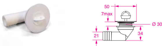
PIEL20F Peso / Weight 21 g cod. 02.10.00011
