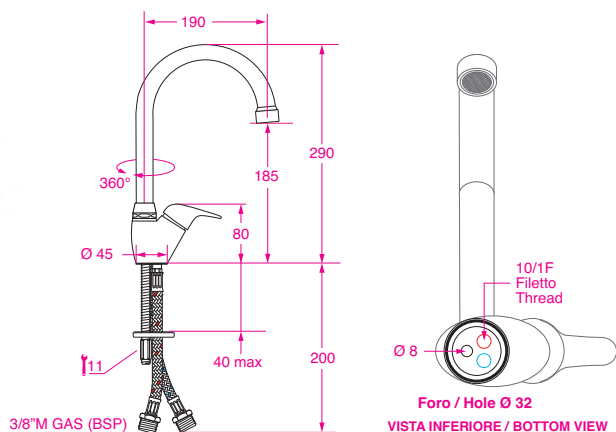
Peso / Weight 1,076 Kg
